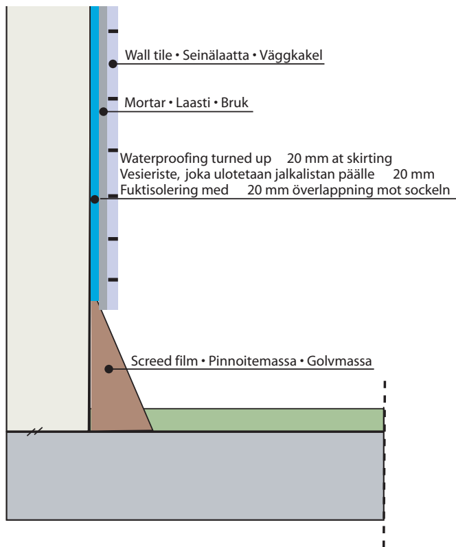
Termination of screed film at skirting. Massapinnoitteen päättäminen jalkalistaan. Anslutning med golvmassa mot sockel.
