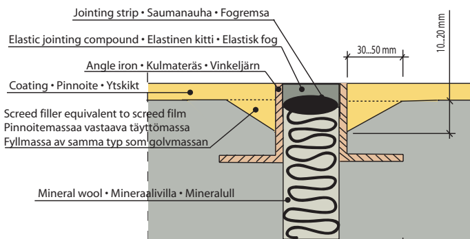
Termination of screed film at expansion joint or equivalent location. Massapinnoitteen päättäminen liikuntasauaman tai vastaavan kohdalla. Anslutning med golvmassa mot rörelsefog eller liknande.
