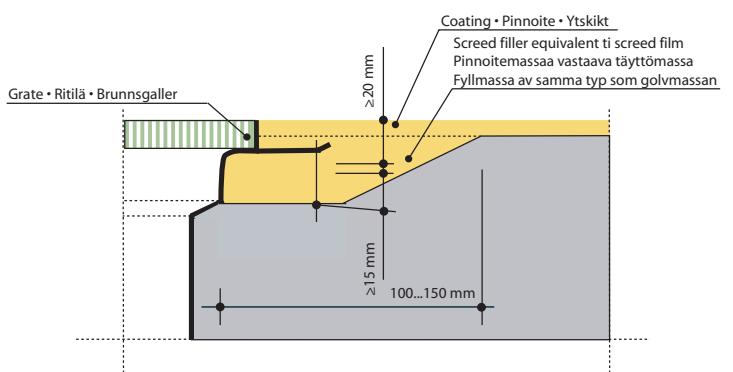
Connection of screed film to floor drain. Massapinnoitteen liittyminen lattiakaivoon. Anslutning med golvmassa mot golvbrunn.
