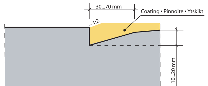
Termination of screed film at continuous concrete surface. Massapinnoitteen päättäminen jatkuvalle betonipinnalle. Anslutning med golvmassa mot betong.
